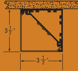
AS350-HO-J AS350-MO-J CEILING MOUNT (FLUSH)
